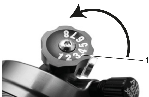
Paveikslėlis 70: „Suntour“ kompresijos reguliatorius ant galinio amortizatoriaus
