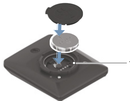
Illustration 148 : Insérer la pile en veillant à la position du joint (1)
