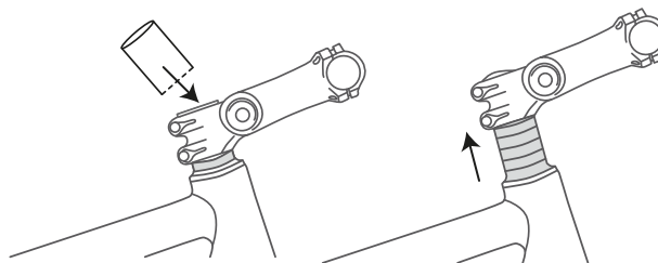
Illustration 120 : Relever la potence Ahead en montant une rondelle d'écartement
