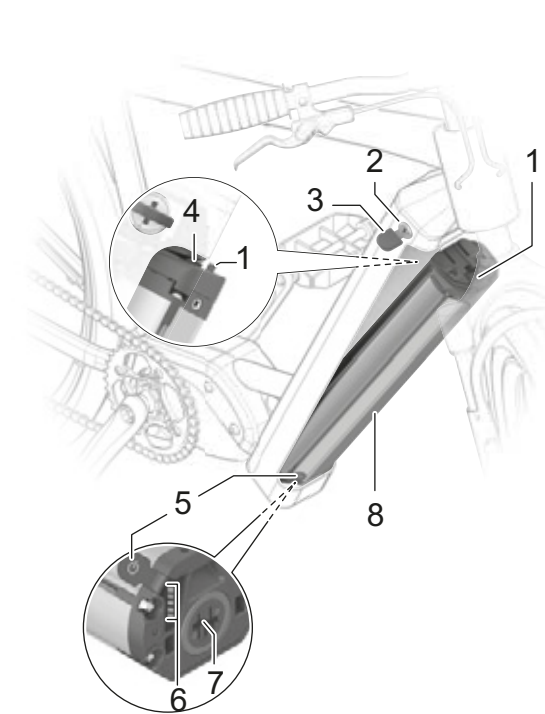
Illustration 49 : Aperçu des variantes de batterie
