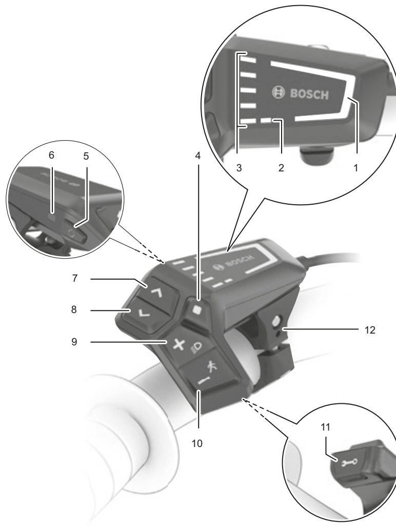
Illustration 54 : Aperçu de l'ordinateur de bord BOSCH LED Remote
