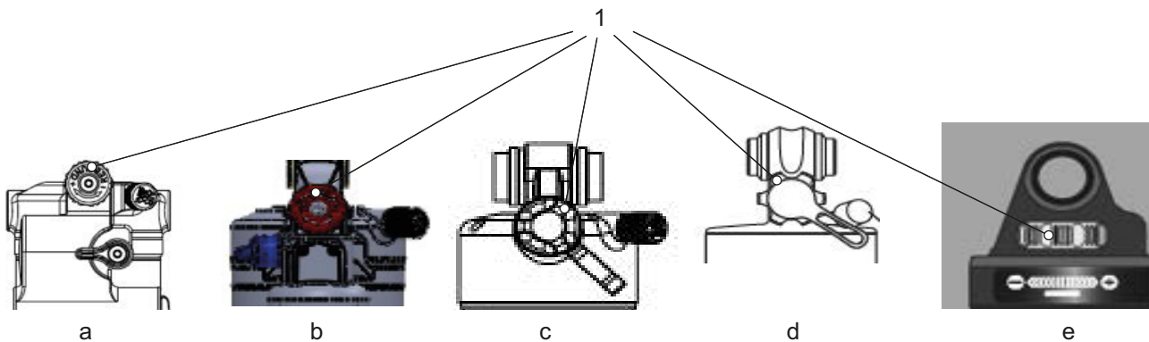
Illustration 228 : Position de la molette de détente SR Suntour sur amortisseur arrière Triair2 (a), Triair (b), EDGE-comp (c), EDGE (d) et RAIDON (e)
