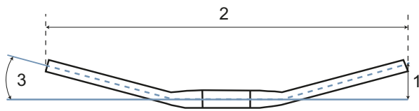
Illustration 11 : Dimensions du guidon
