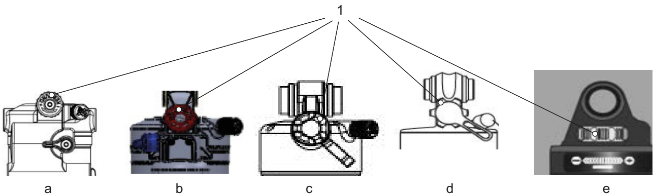
Illustration 226 : Position de la molette de détente SR Suntour sur amortisseur arrière Triair2 (a), Triair (b), EDGE-comp (c), EDGE (d) et RAIDON (e)
