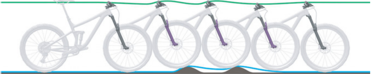
Illustration 221 : Détente trop lente de la fourche suspendue
