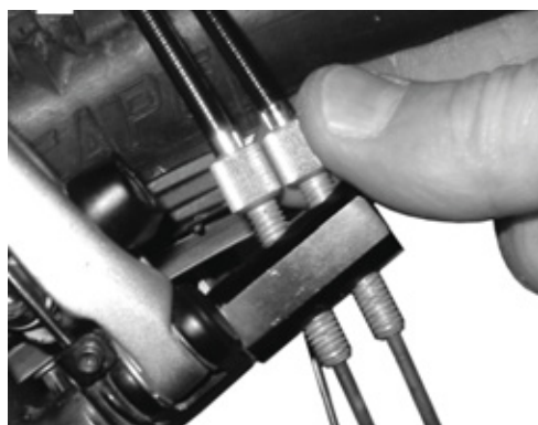
Illustration 211 : Sur les versions de moyeux ROHLOFF avec commande interne du changement de vitesse, le dispositif de réglage de la tension est situé sur le contre-support de tension.
