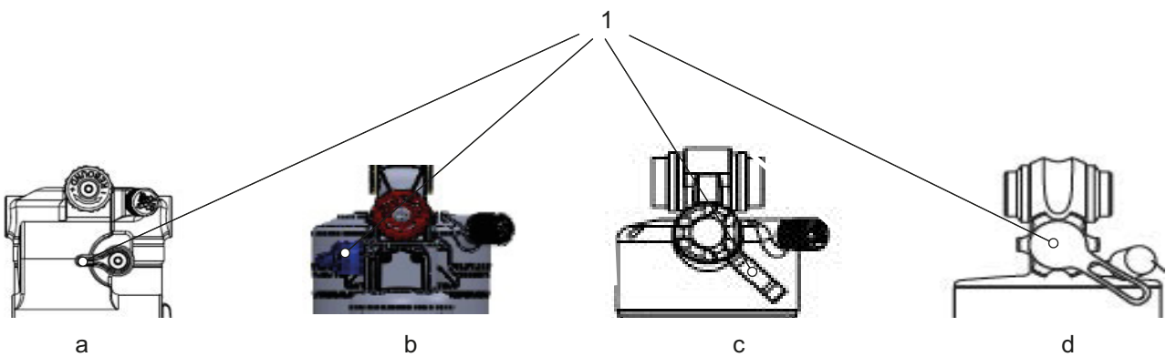
Illustration 232 : Position du levier de compression SR Suntour sur amortisseur arrière Triair2 (a), Triair (b), EDGE-comp (c), EDGE (d)
