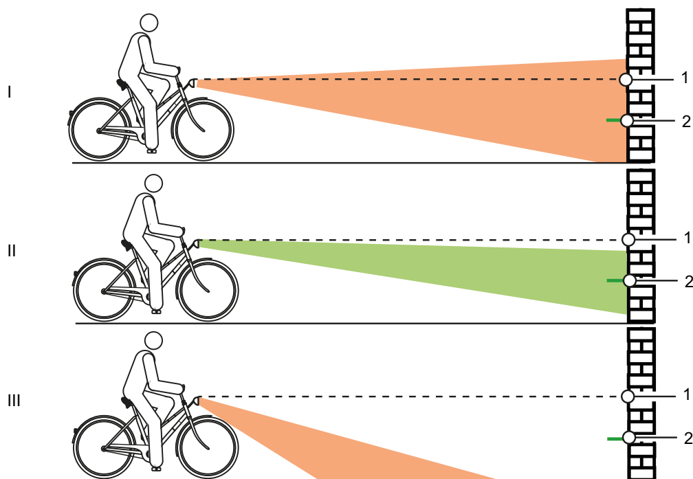
Illustration 209 : Feu réglé trop haut (1), correctement (2) et trop bas (3)
