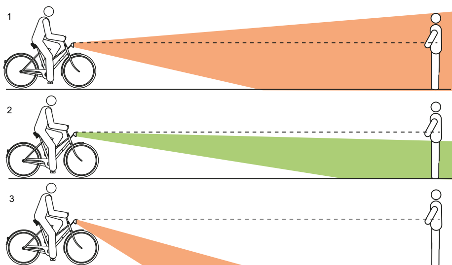
Illustration 144 : Feu réglé trop haut (1), correctement (2) et trop bas (3)
