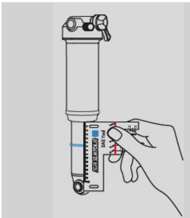
Illustration 139 : Mesurer la course de suspension totale
