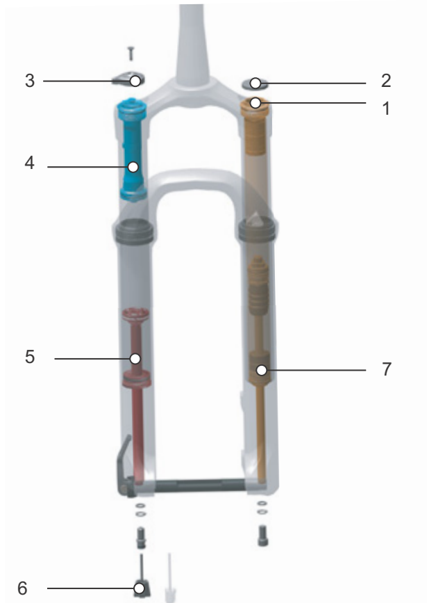
Illustration 14 : Structure interne de la fourche de suspension pneumatique
