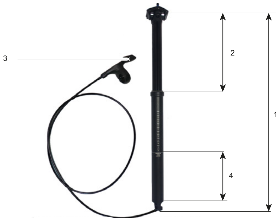
Illustration 40 : Structure et dimensions de la tige de selle LIMOTEC A1
