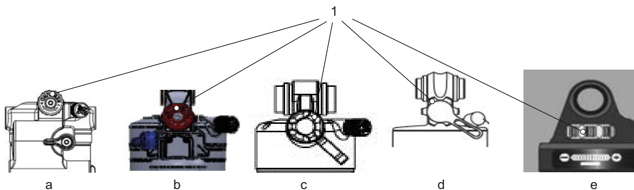
Illustration 143 : Position de la molette de détente SR Suntour sur amortisseur arrière Triair2 (a), Triair (b), EDGE-comp (c), EDGE (d) et RAIDON (e)
