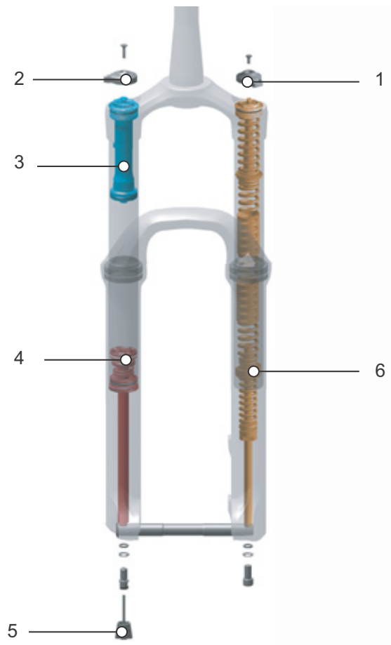
Illustration 15 : Structure interne de la fourche à ressort en acier
