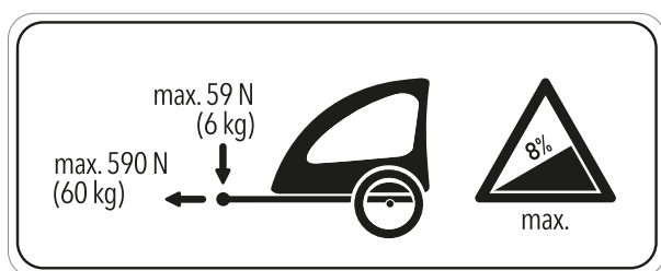
Illustration 153 : Plaque d'information de la remorque
