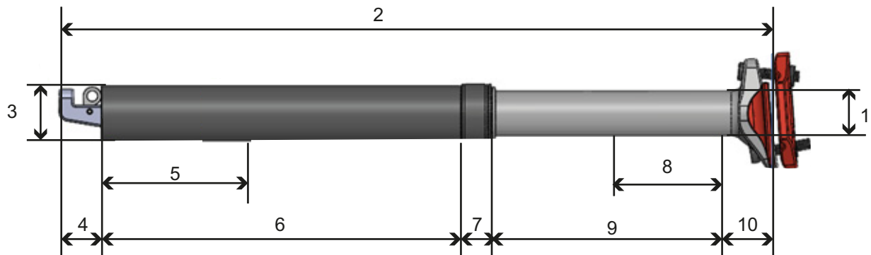
Illustration 63 : Poids de la tige de selle LIMOTEC, A3/A3 Plus
