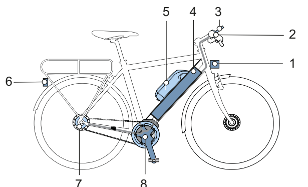
Illustration 48 : Schéma du système d'entraînement électrique avec composants électriques
