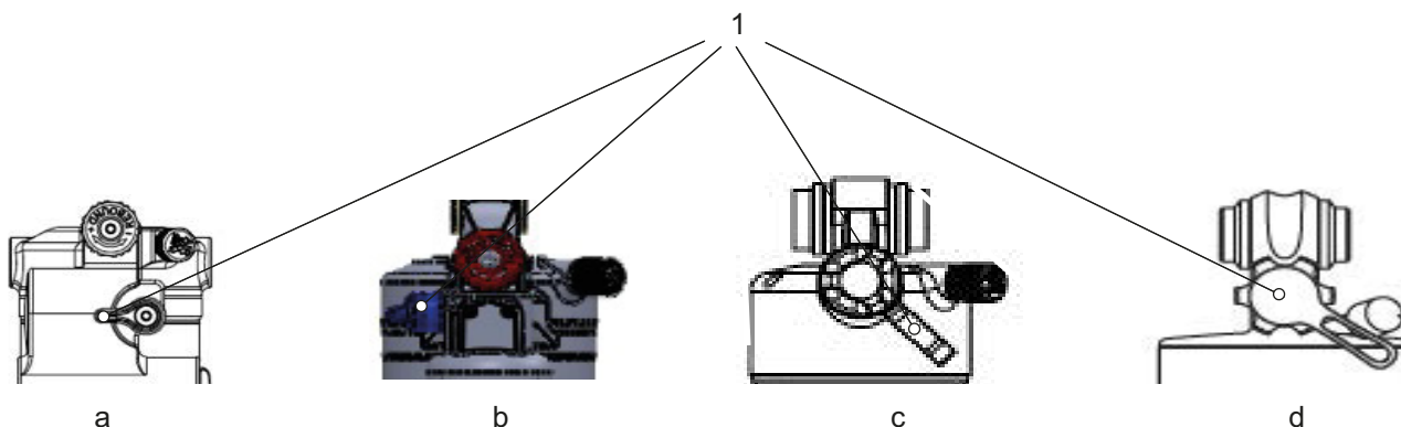
Illustration 166 : Position du dispositif de réglage de la compression SR Suntour sur amortisseur arrière Triair2 (a), Triair (b), EDGE-comp (c), EDGE (d)
