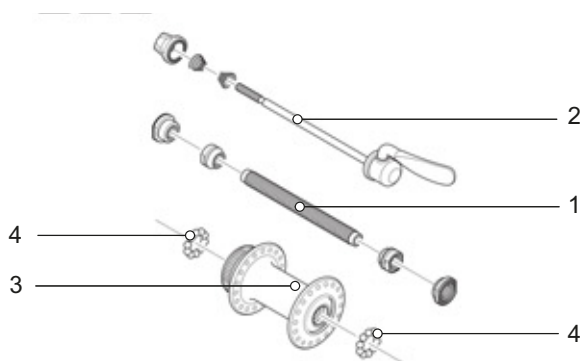
Illustration 32 : Exemple d'un moyeu de roue avant, SHIMANO
