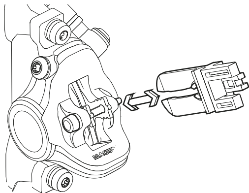
Illustration 66 : Insérer la cale de transport
