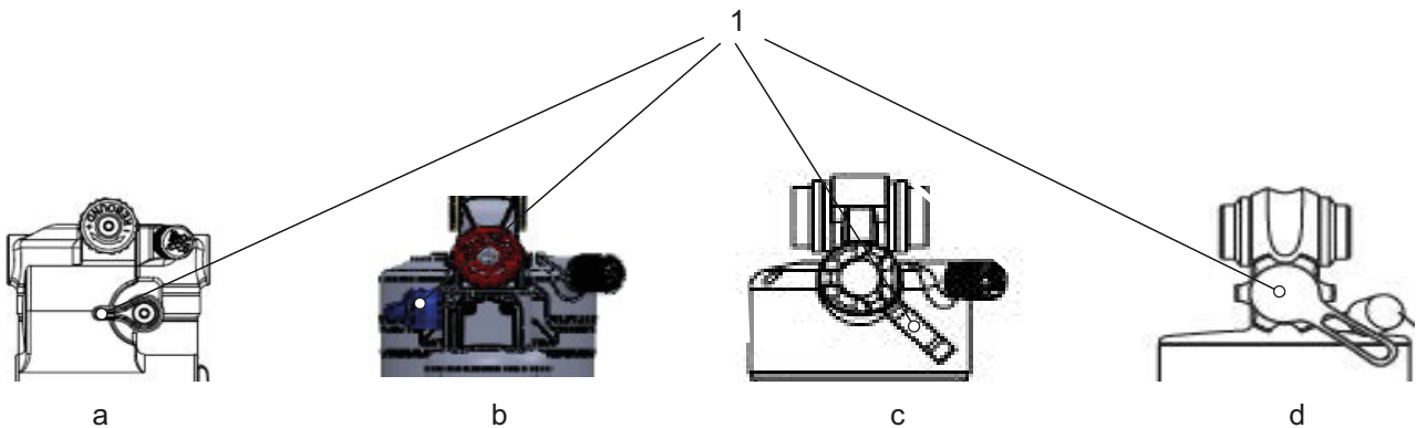
Illustration 230 : Position du levier de compression SR Suntour sur amortisseur arrière Triair2 (a), Triair (b), EDGE-comp (c), EDGE (d)
