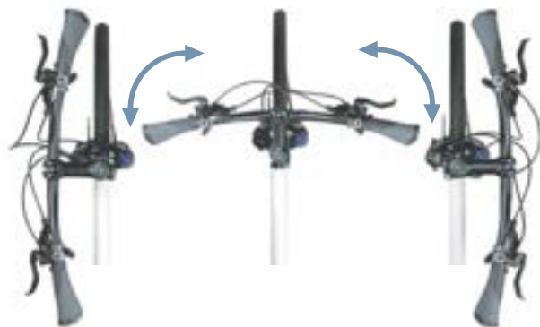
Illustration 10 : Fonction Twist, exemple d'un BY.SCHULZ
