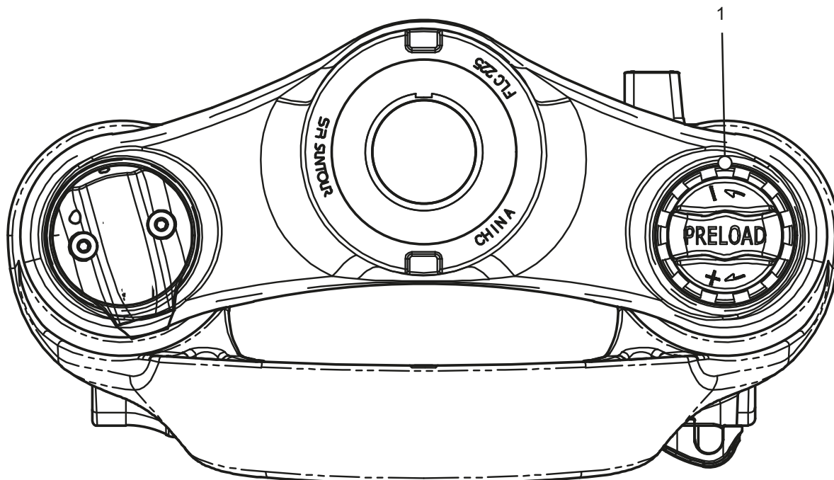
Illustration 134 : Exemple d'une SR SUNTOUR, molette de réglage du sag sur la couronne de fourche
