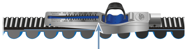
Illustration 203 : Gabarit de contrôle sur la courroie
