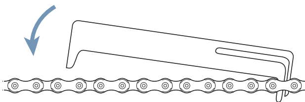
Illustration 195 : Abaisser le gabarit de mesure à gauche
