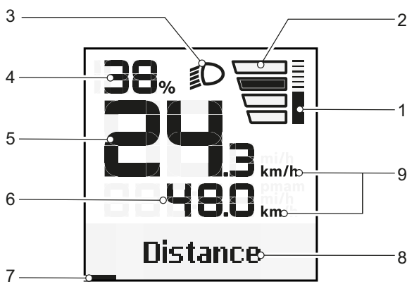
Illustration 56 : Aperçu de l'écran de départ
