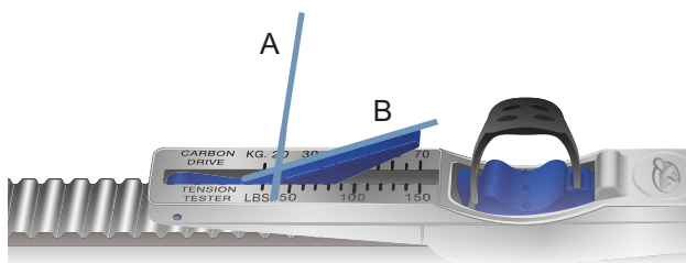
Illustration 205 : Exemple de valeur indiquée : 20 kg
