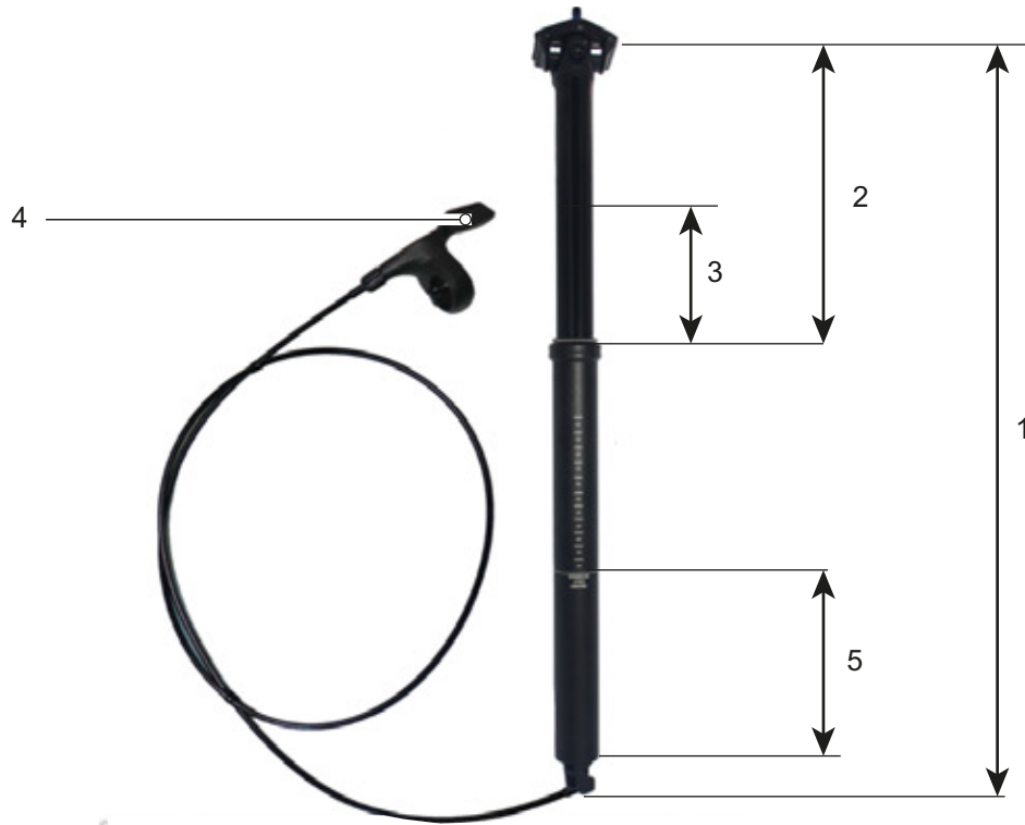
Illustration 41 : Structure et dimensions de la tige de selle LIMOTEC Alpha 3
