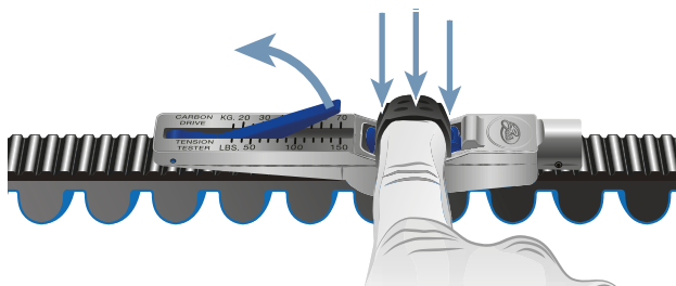
Illustration 204 : Abaisser le gabarit de contrôle avec un doigt
