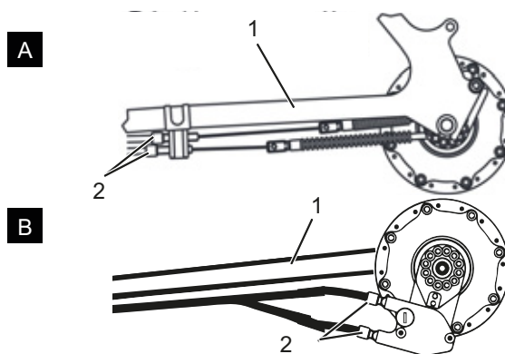
Illustration 213 : Douilles de réglage (2) sur deux modèles alternatifs (A et B) d'un changement de vitesse actionné par câble à deux câbles sur la base de cadre (1)
