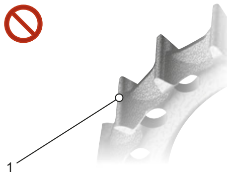
Illustration 200 : Profil de cran usé
