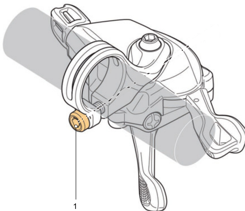
Illustration 130 : Position de la vis de fixation du levier de vitesse SHIMANO (1)
